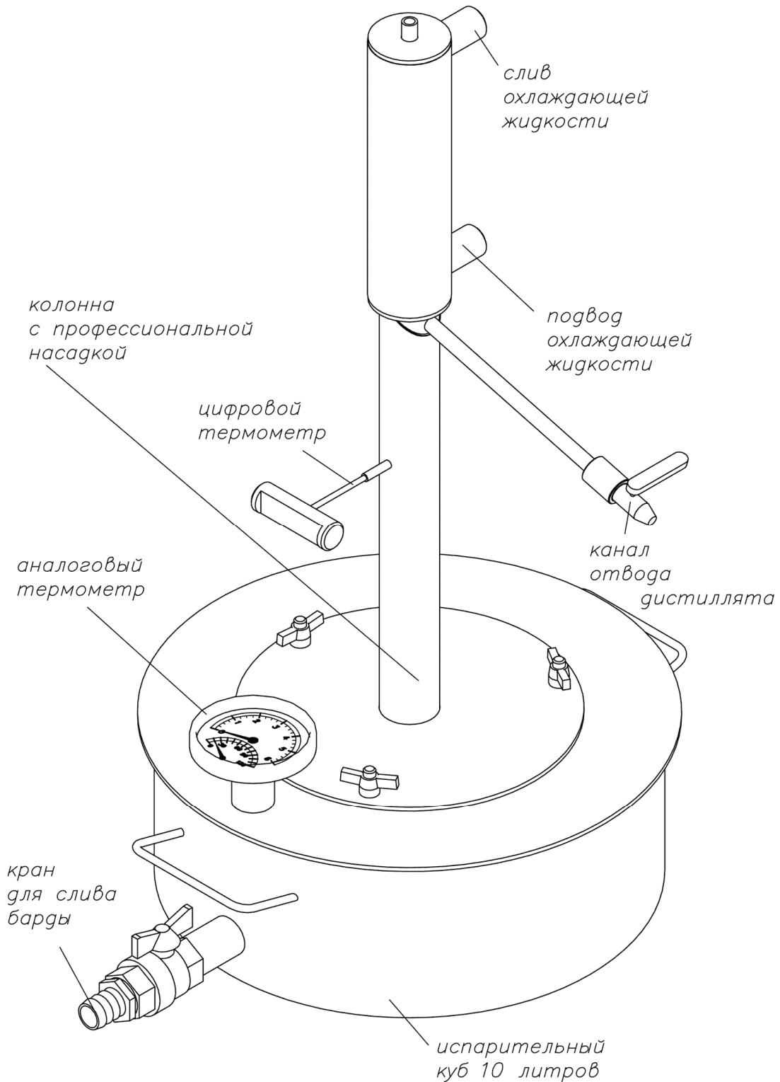
Рис 1. Мини спирт завод модель «миджет».
